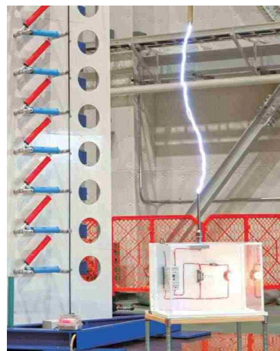
高電圧試験設備での放電実験の様子。雷の電圧を模擬的に再現し、得られたデータを製品開発などに生かしています。
